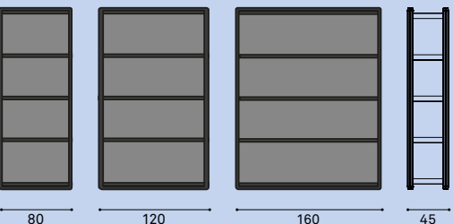
shelves with upholstered panel - depth 38 cm / Ablagen mit gepolstertem Paneel - 38 cm tief
