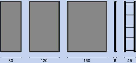
acoustic panel upholstered - single- or double sided / Akustisches Paneel - ein- oder doppelseitig gepolstert
