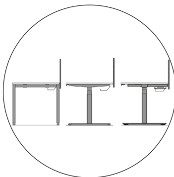
Übersicht Motion - Flux E - Flux E Plus mit Noova Desk Panel Pure
