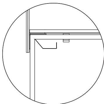
Seitenansicht Montage Noova Desk Panel Pure
